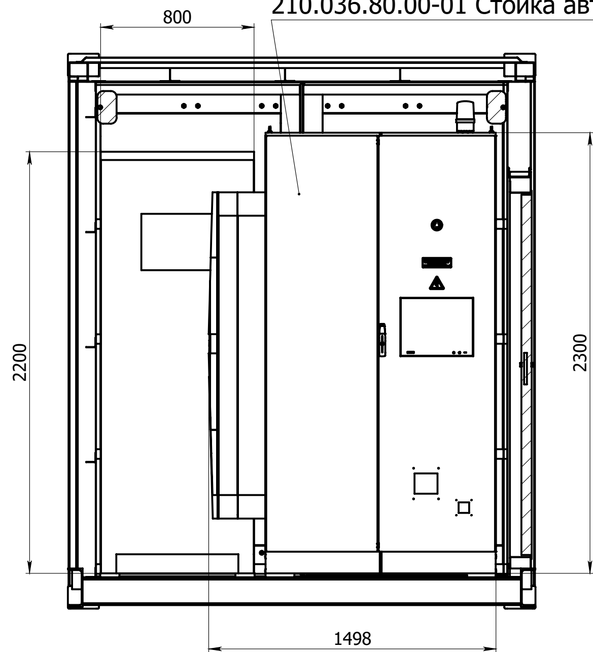
Б-Б 210.036.80.00-01 Стойка автоматического управления
