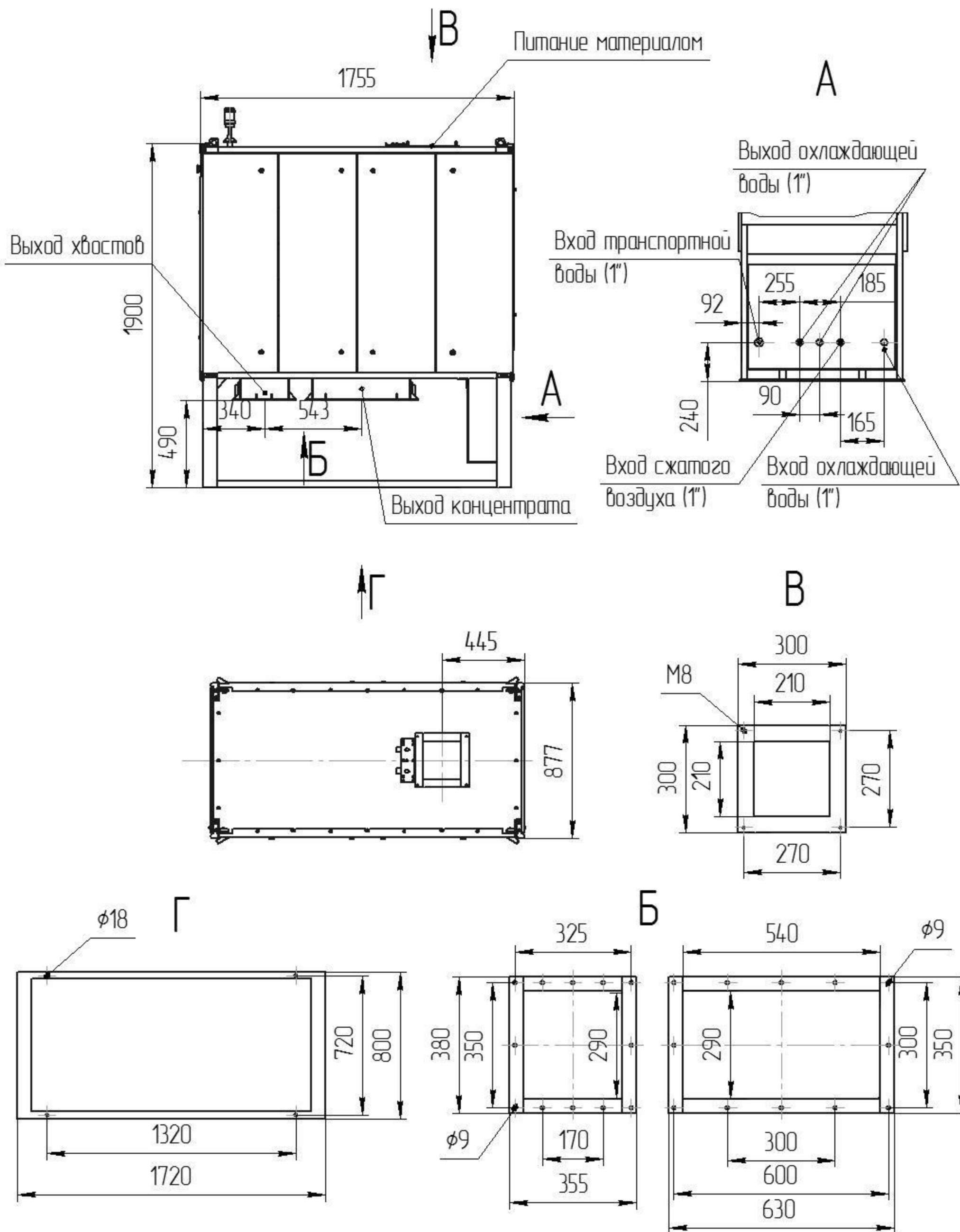
Машина сортировочная ЛС-ОД-50-04
