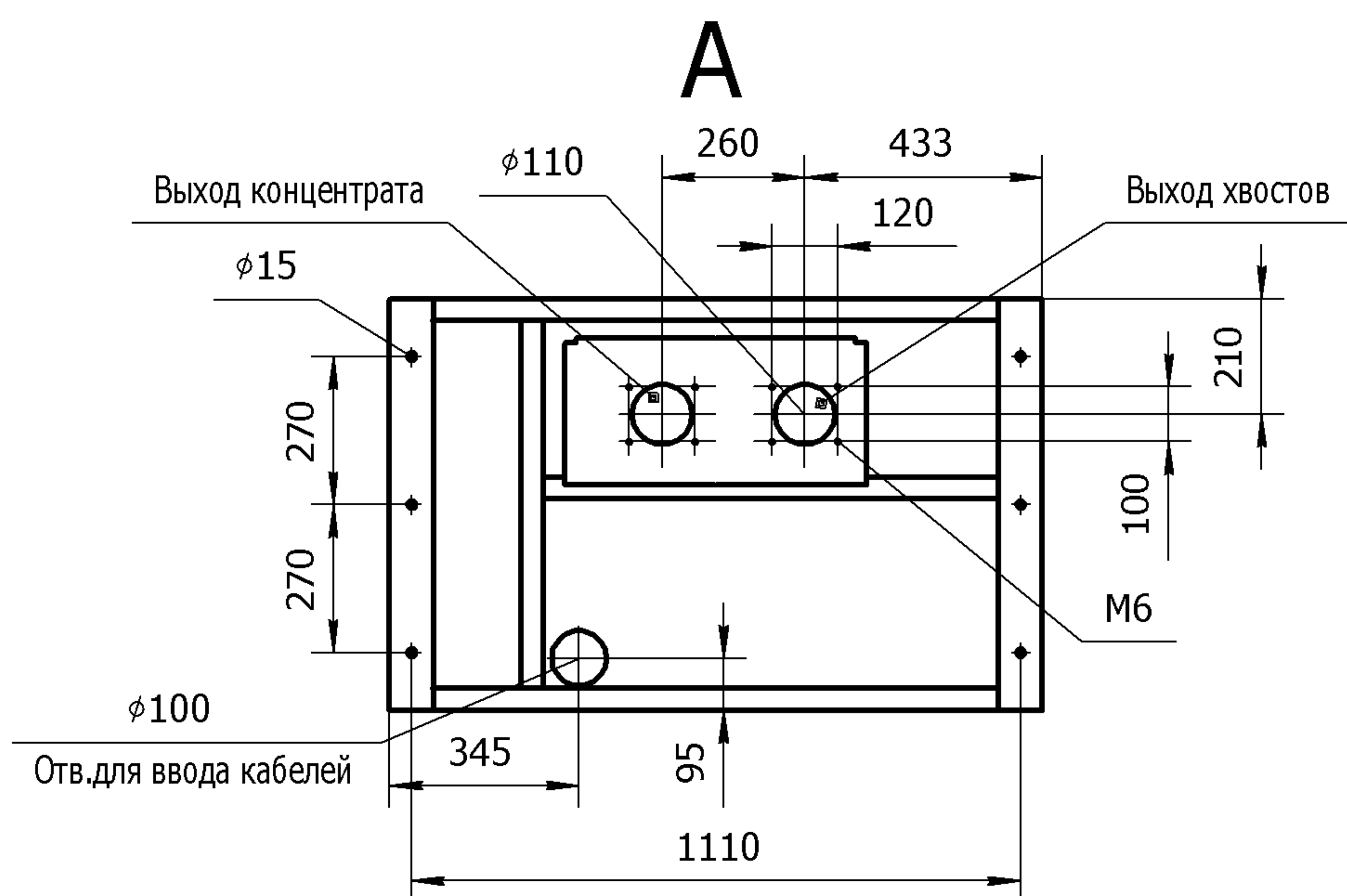
Машина сортировочная ЛС-Д-4-03П
